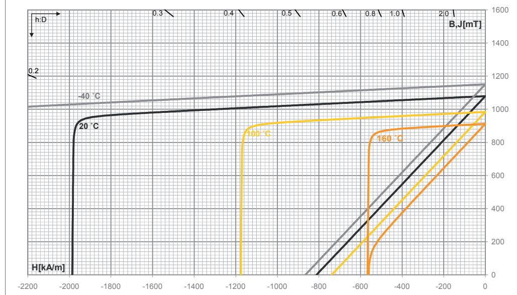
Entmagnetisierungskurve
